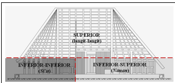
Gambar 20. Organisasi ruang vertikal Sonaf Nis None (Sumber: Dokumentasi Pribadi, 2015)
