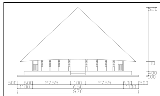
Gambar 3. Tampak depan Sonaf Nis None (Sumber: Dokumentasi Pribadi, 2015)
