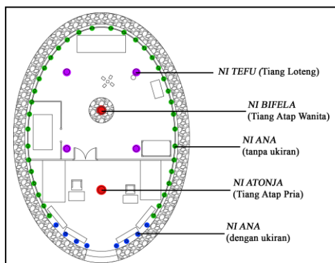
Gambar 25. Tata letak tiang pada Sonaf Nis None (Sumber: Dokumentasi Pribadi, 2015)
