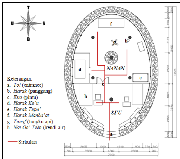
Gambar 14. Denah Sonaf Nis None (Sumber: Dokumentasi Pribadi, 2015)
