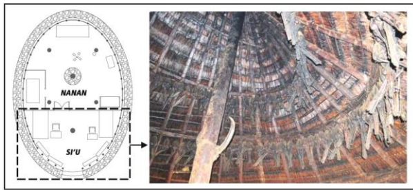
Gambar 23. Langit-langit pada si'u Sonaf Nis None (Sumber: Dokumentasi Pribadi, 2015)
