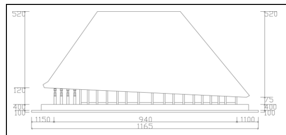
Gambar 4. Tampak samping Sonaf Nis None (Sumber: Dokumentasi Pribadi, 2015)
