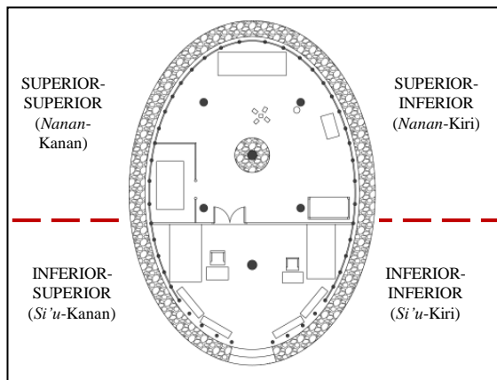
Gambar 19. Organisasi ruang horisontal Sonaf Nis None (Sumber: Dokumentasi Pribadi, 2015)
