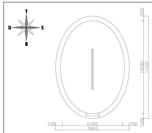
Gambar 2. Tampak atas Sonaf Nis None (Sumber: Dokumentasi Pribadi, 2015)
