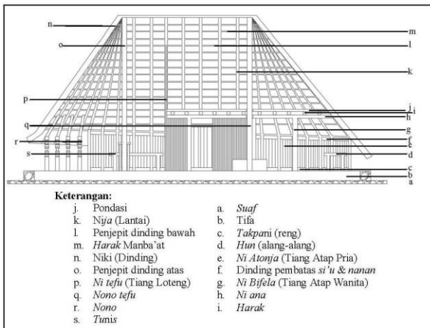
Gambar 41. Potongan Sonaf Nis None (Sumber: Dokumentasi Pribadi, 2015)
