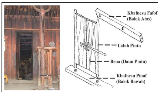
Gambar 31. Enok (pintu) Sonaf Nis None [1]
